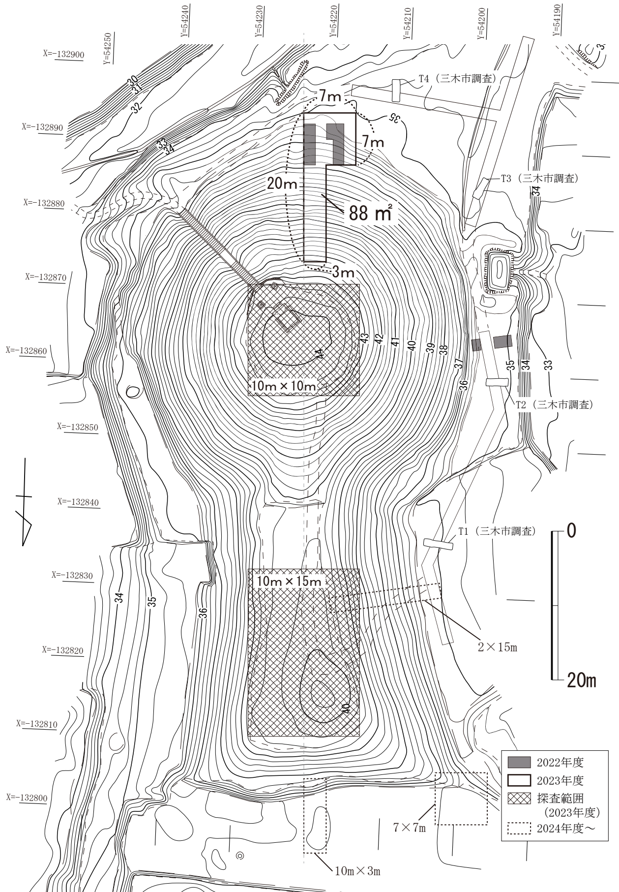
図2 三木市愛宕山古墳 調査区配置図
