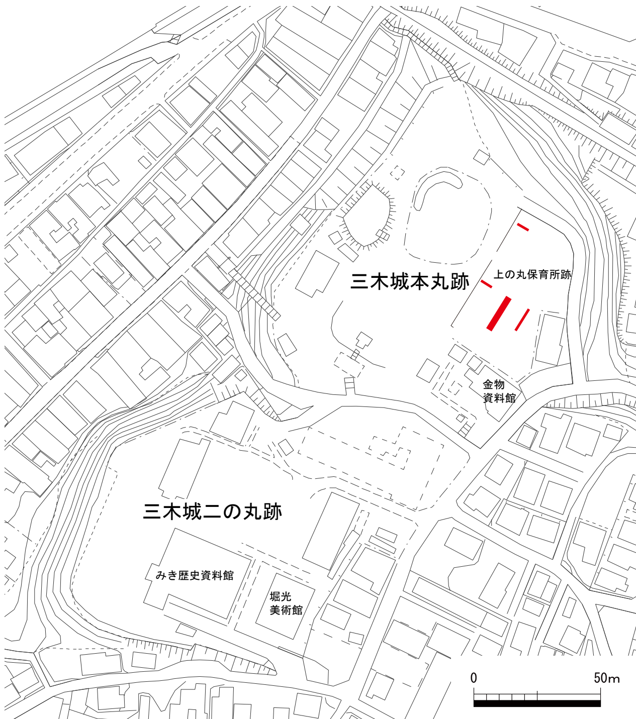
三木城本丸跡 調査区配置図（予定）
