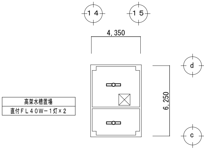
P H 階 平面図
