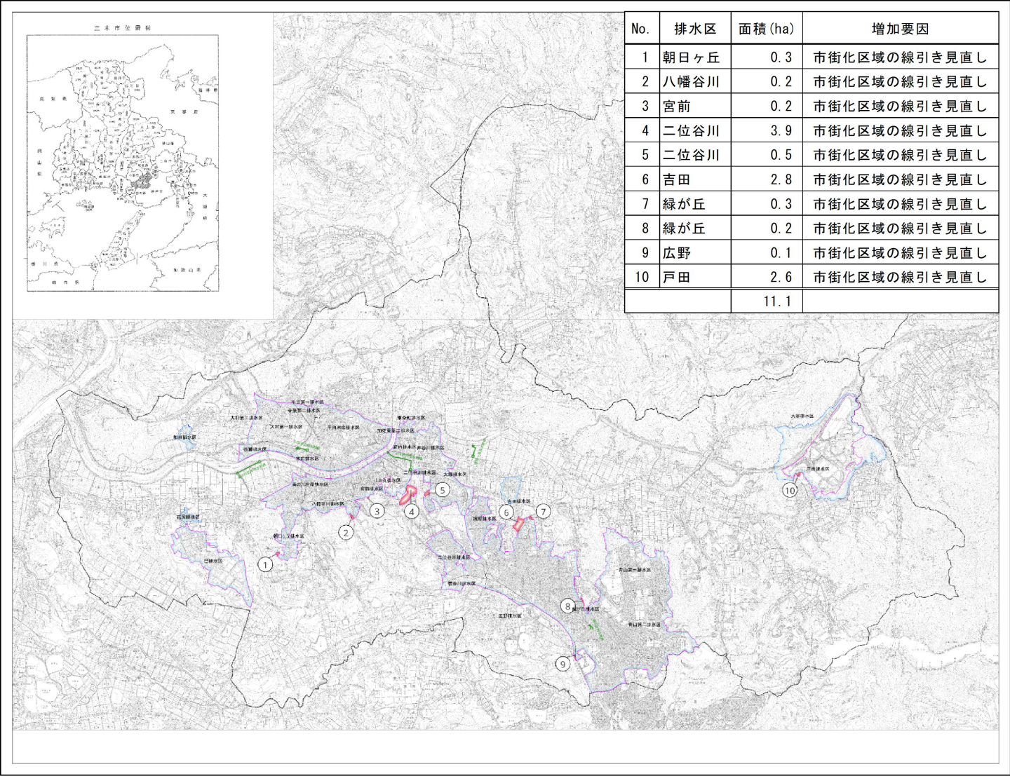
総 括 図（雨水）
